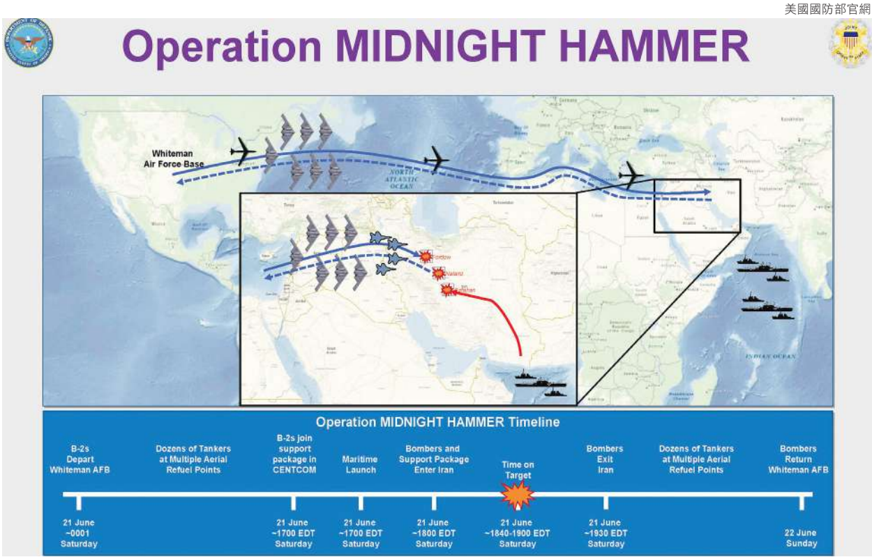
美國於6月22日凌晨展開代號「午夜之錘」空襲。圖為美軍公布之攻擊路徑與時序圖。
